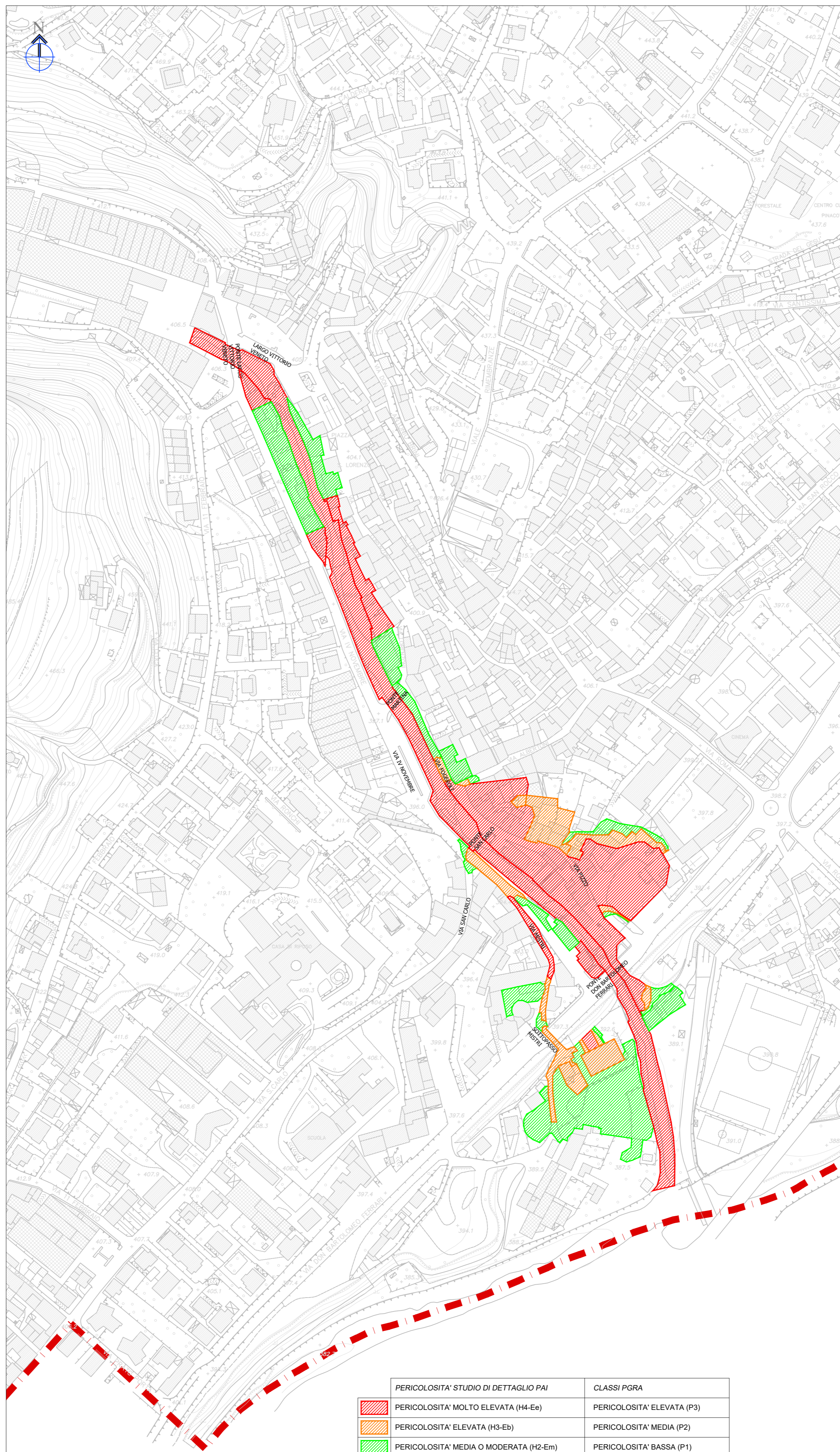
PLANIMETRIA ZONE DI PERICOLOSITA' - SINOTTICA CRITERI MORFOLOGICI E IDRAULICI Scala 1:2000
