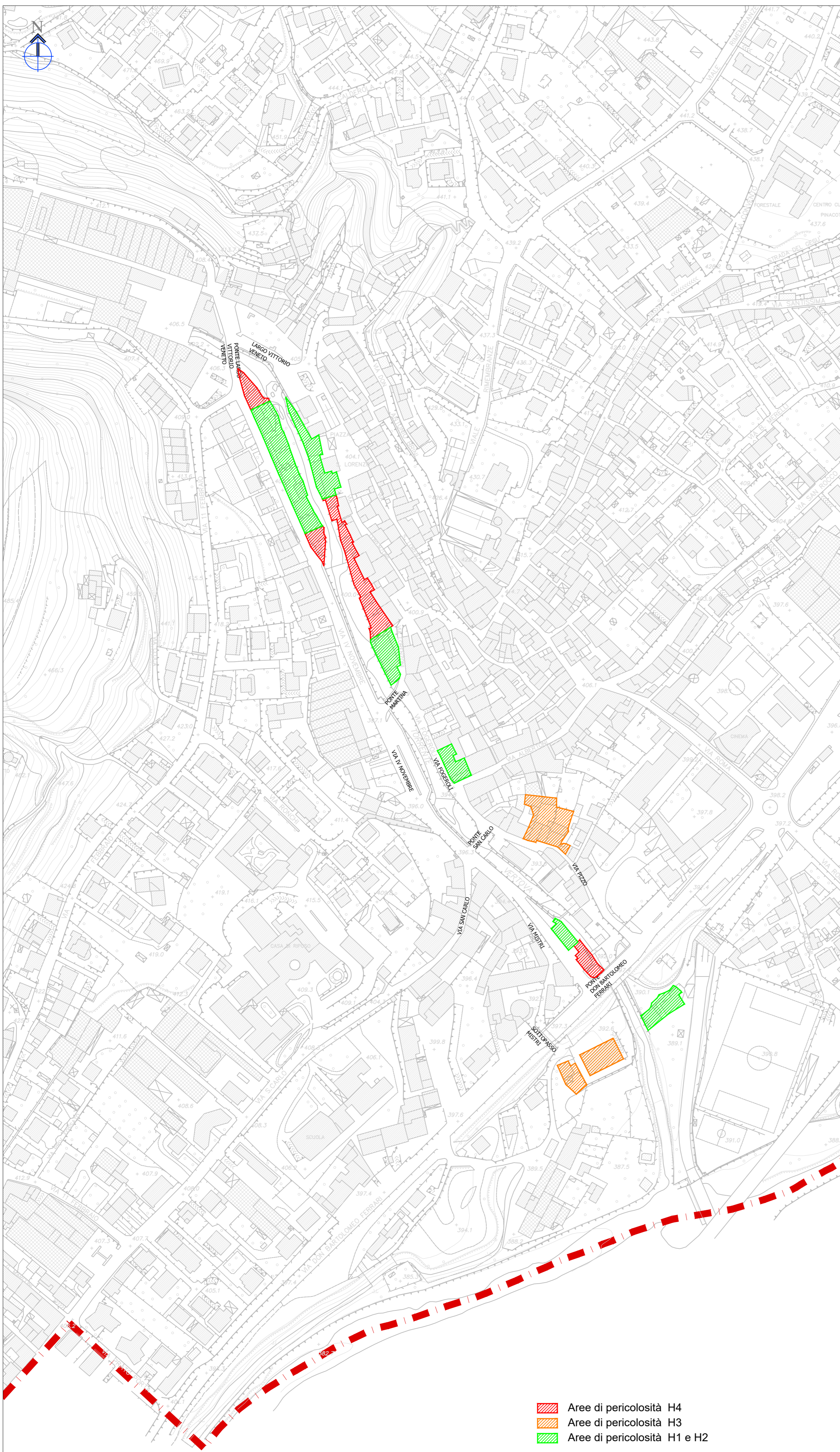
PLANIMETRIA ZONE DI PERICOLOSITA' DA CRITERI MORFOLOGICI Scala 1:2000
